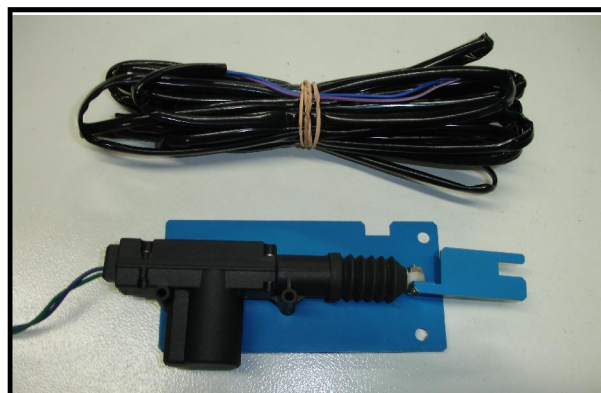
Foto A Demonstrativo do Kit Suporte para Trava Elétrica
